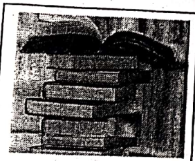
۸ جلد کتاب
