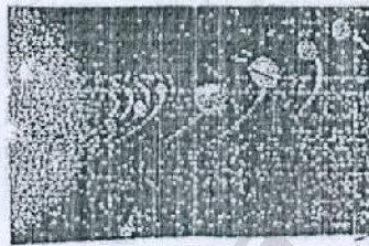
(c) سیارات
