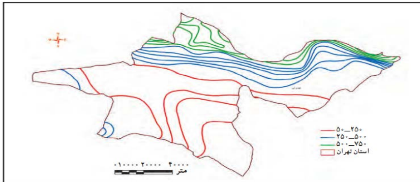
شکل ۹-۱- نقشه هم‌بارش استان تهران
